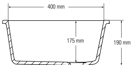
Boční řez
