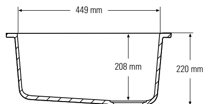
Boční řez
