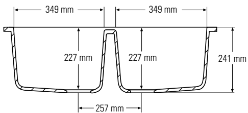
Přední řez
