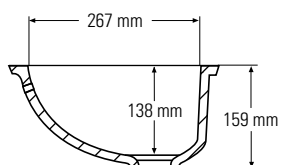
Boční řez
