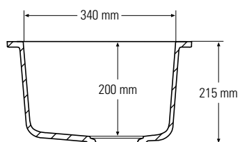
Boční řez
