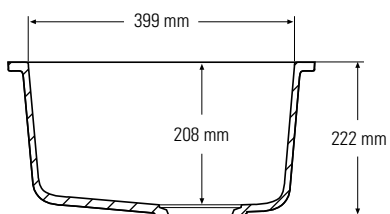
Boční řez
