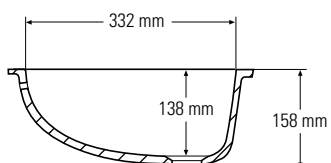
Boční řez
