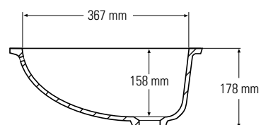
Boční řez
