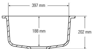
Boční řez
