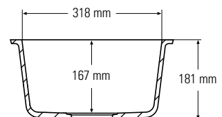
Boční řez
